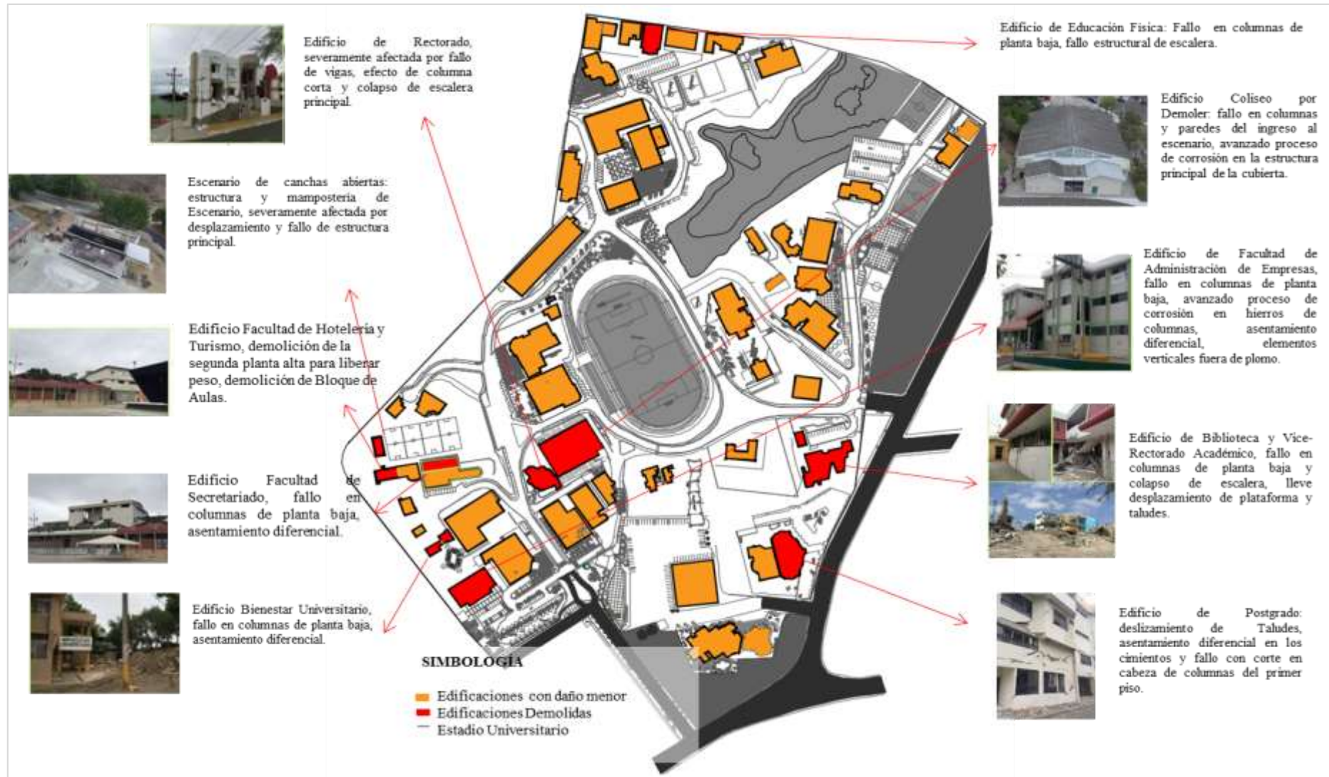
Figura 12: Afectaciones post-terremoto 16A Fuente: Observatorio Territorial – Facultad de Arquitectura
